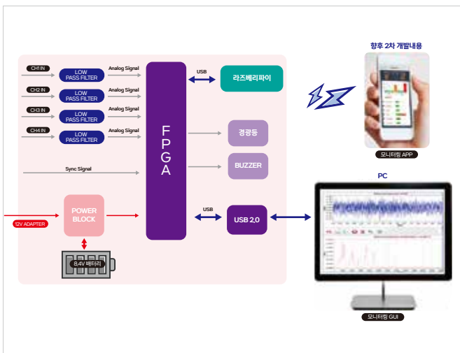
FPGA를 이용한 고속 샘플링 모니터링
